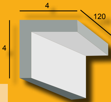
canal 4x4x120 CO44
