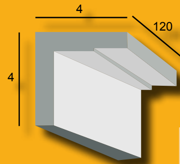
canal rebajado 4x4 x120 CO44R
