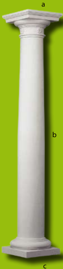
dórica estrada D205 opción dórica lisa DL205 Ø22 a: 34 b: 205 c: 34
